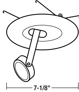
Trim OD: 7-1/8"
