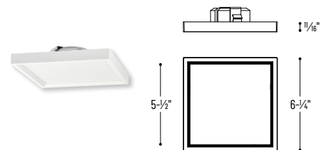
NLOS-S62L 6" Square SURF
