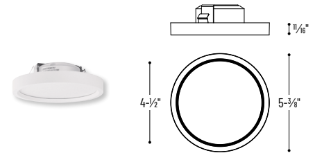
NLOS-R42L 4" Round SURF
