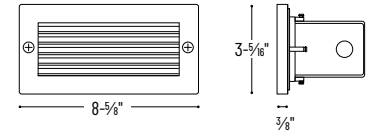
NSW-851/32 Louver
